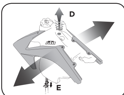
4. Rimuovere il rubinetto, rimuovere i fianchetti, rimuovere la vite-sella Remove the petcock, remove the radiator scoops, remove the seat screw
