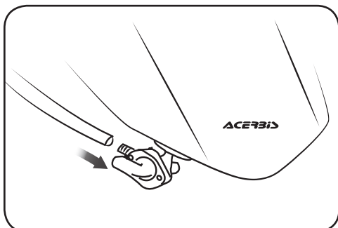
6. Riposizionare il tubo Attach the fuel line
