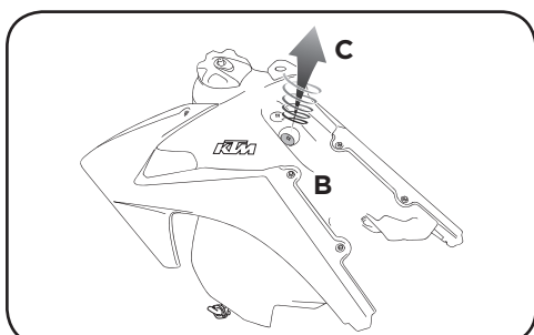
3. Svitare la vite serbatoio e rimuovere il serbatoio Unscrew the tank screw and remove the tank
