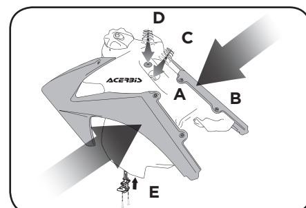
5. Posizionare il serbatoio acerbis. Montare il rubinetto (torque spec: 1,8ft/lb 2,5N/m). Rimettere la vite sella. Montare i fianchetti. Rimettere la vite-serbatoio Place the acerbis tank. Install the petcock (torque spec: 1,8ft/lb 2,5N/m). Install the seat screw. Attach the radiator scoop. Install the tank screw
